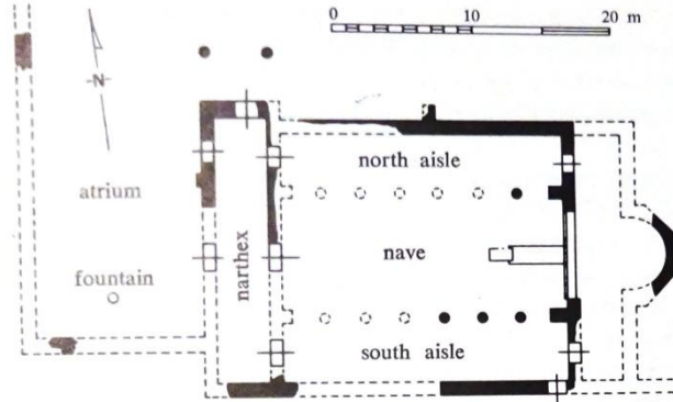
La basilique du Saray, plan au sol
