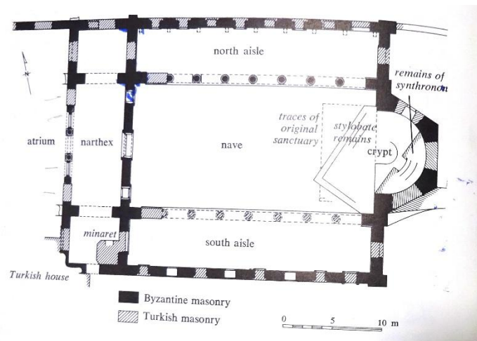
La basilique du Saray, plan au sol
